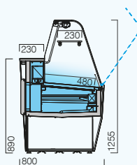
VPRTRE - VC vitrina serve-over counter 3M2 (-1... +7 °C) DIM. 980 | 1280 | 1480 1880 | 2480
