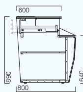
CXPRT caixa support case DIM. 680
